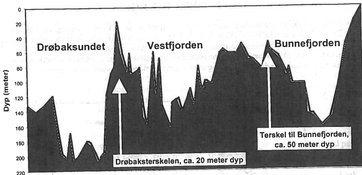
Figur 2. Langsgående dybdeprofil av indre Oslofjord fra Bunnefjorden til Drøbaksundet.
