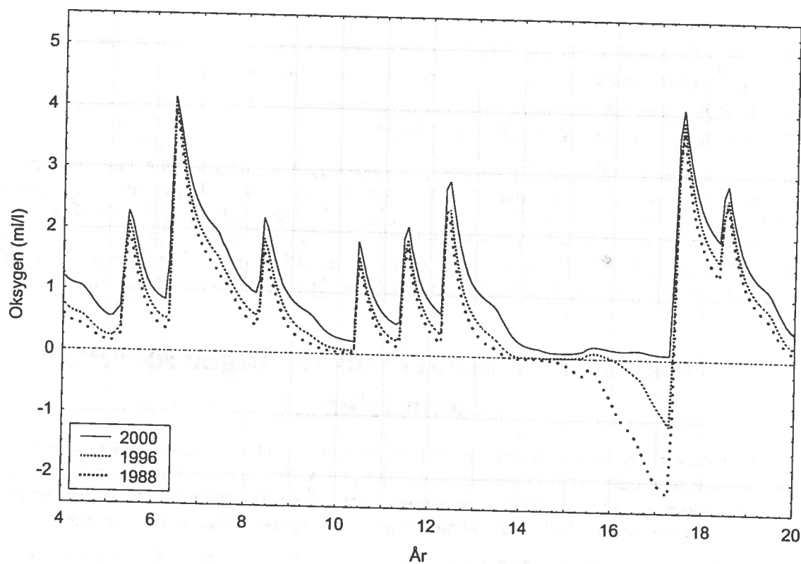
Figur 9. Oksygenkonsentrasjon i Bunnefjorden på 80 m dyp for to historiske og en aktuell utslippssituasjon.
