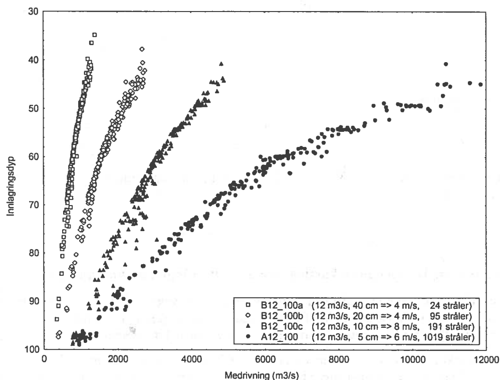
Figur 20. Innlagringsdyp mot medrivning beregnet for nedpumping av 12 m 3 /s til 100 m dyp, for scenarier med ulik strålediameter og -hastighet.
