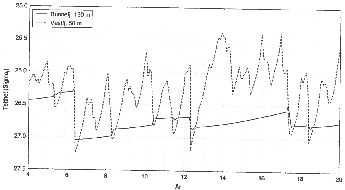
Figur 11. Variasjon i tetthet i dypvannet i Bunnfjorden og i Vestfjorden på terskeldypet mellom de to bassengene for utslipps-scenario 2000. Legg merke til at vertikal akse er snudd, slik at tettheten øker nedover.
