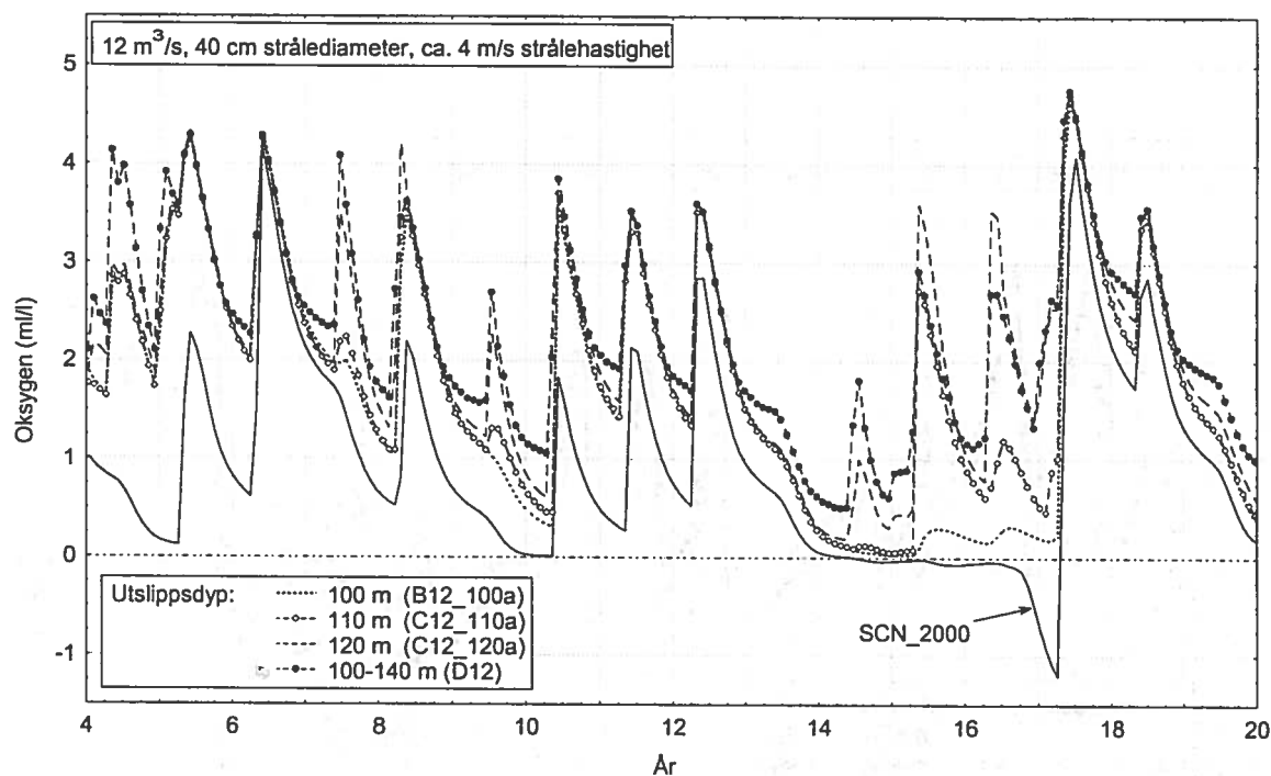
Figur 22. Oksygen på 130 m dyp i Bunnefjorden ved pumping av 12 m 3 /s i stråler med 40 cm diameter og med utgangshastighet 4 m/s, ved ulike utslippsdyp. Scenario 2000 er tatt med som sammenligningsgrunnlag.
