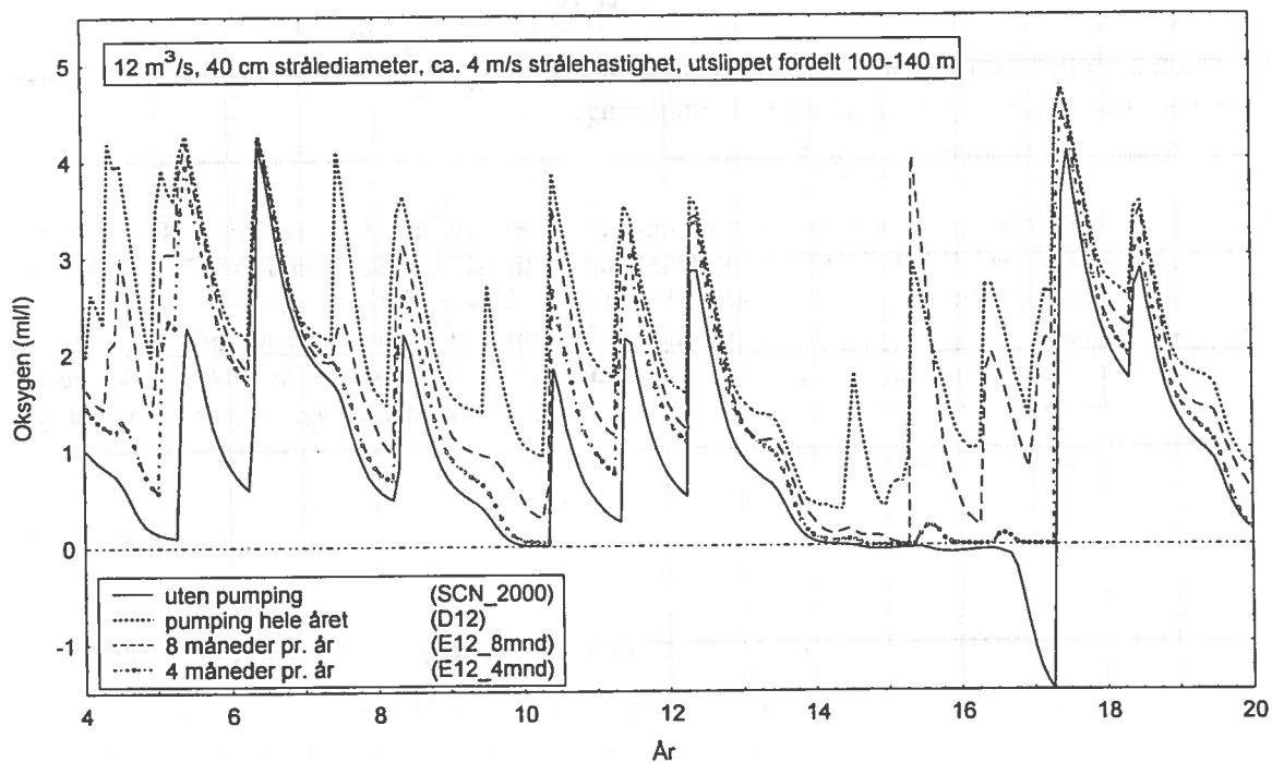
Figur 26. Simulert oksygenkonsentrasjon på 143 m dyp i Bunnefjorden for scenarier med fast sesongbegrensning avpumpeperioden, sammenlignet med situasjon uten pumping og med pumping hele året. Utslipet fordelt 100-140 m. Scenario 2000 er tatt med som sammenligningsgrunnlag.
