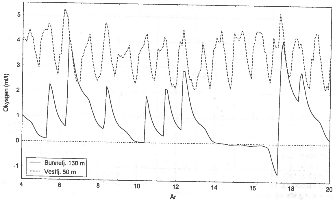
Figur 12. Oksygenkonsentrasjoner i Bunnfjorden på 130 m dyp og i Vestfjorden på terskeldypet (50 m) mellom de to bassengene for utslipps-scenario 2000.
