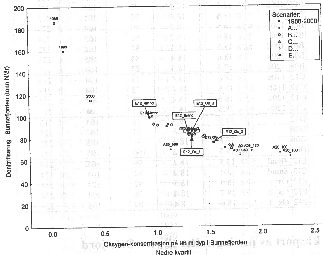
Figur 30. Denitrifisering i Bunnefjorden mot oksygenforhold i dypvannet i det samme bassenget for ulike scenarier. Scenarie-betegnelser er angitt for hvert punkt.
