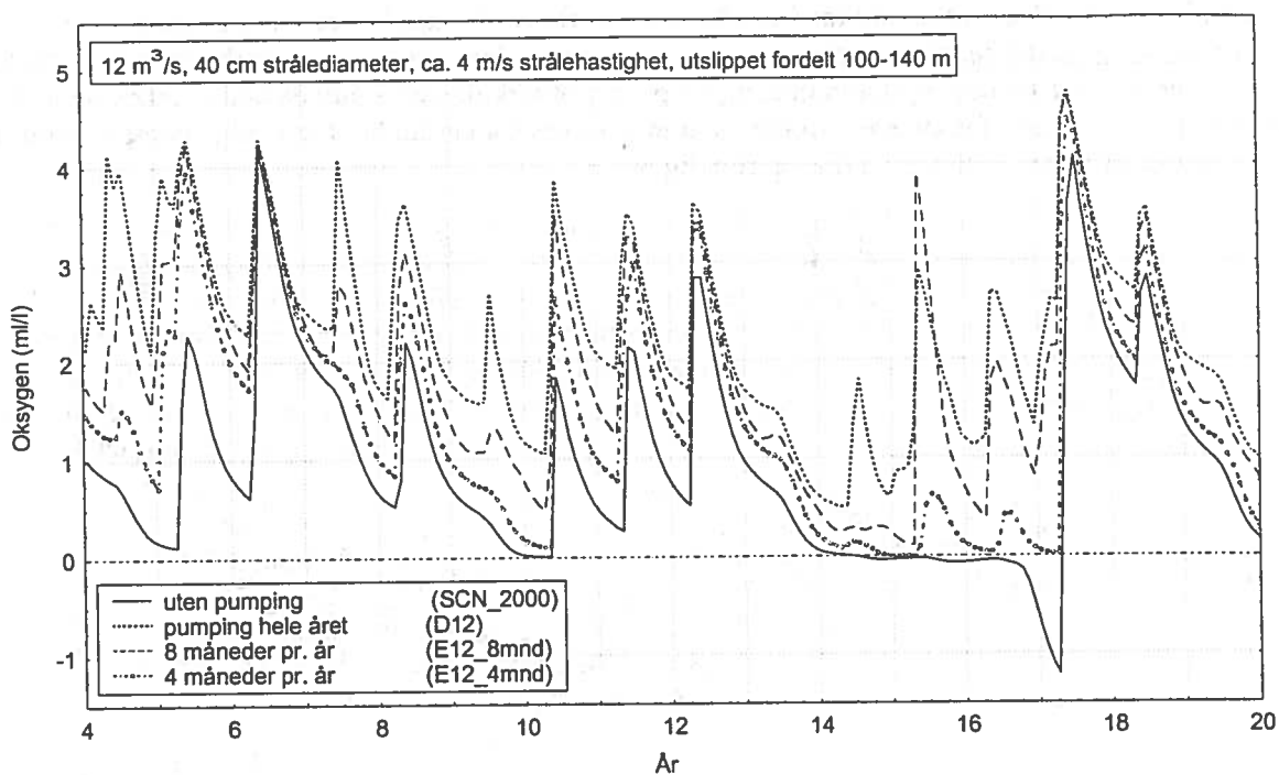
Figur 25. Simulert oksygenkonsentrasjon på 130 m dyp i Bunnefjorden for scenarier med fast sesongbegrensning avpumpeperioden, sammenlignet med situasjon uten pumping og med pumping hele året. Utslipet fordelt 100-140 m.
