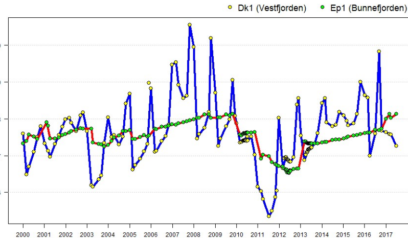
Temperaturutvikling (2000-2017) ved 90 meters vanddyb i stasjon Dk1 (Vestfjorden) og 80 meters vanddyb i stasjon Ep1 (Bunnefjorden). * Data 2000-2014 Niva og 2015-2017 Norconsult
